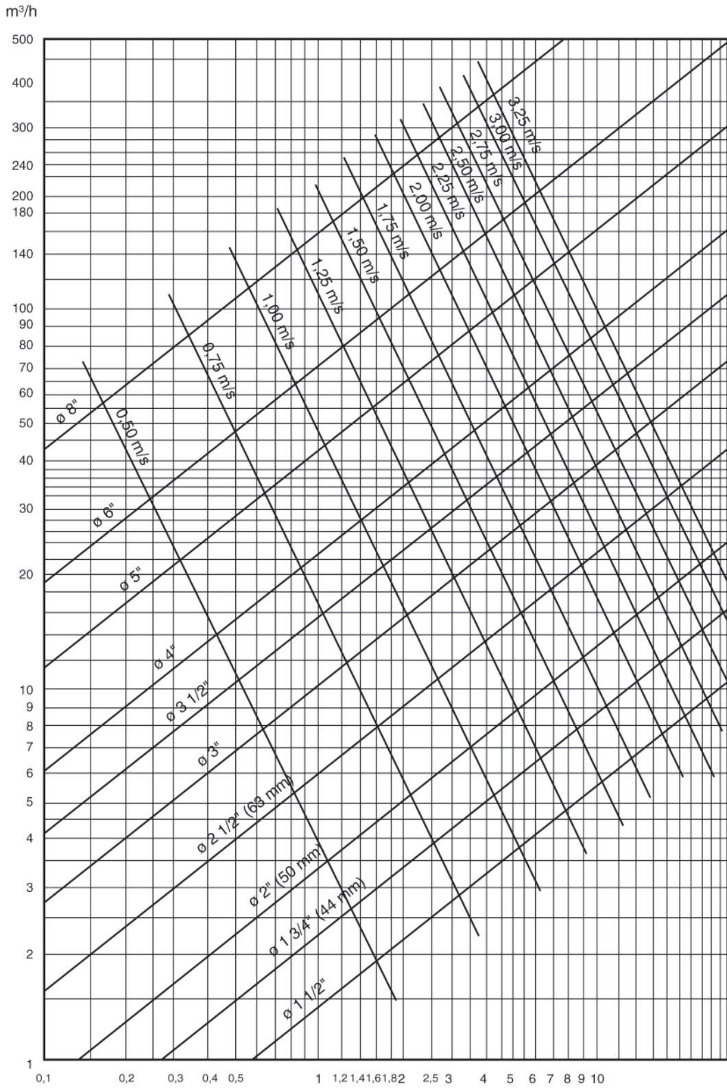
PÉRDIDA DE CARGA EN m. X 100 m. DE TUBERÍA Los gráficos reflejan las pruebas con tubos de 6m. de longitud. LOST OF LOAD ON m x 100 OF PIPING PERTES DE CHARGE EN m x 100 MTS.
