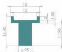
CALZO MARCO Corte Recto
